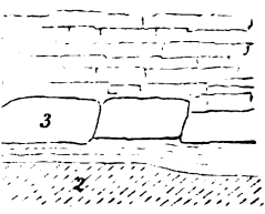
neisskeiles am Gstellhorn.
